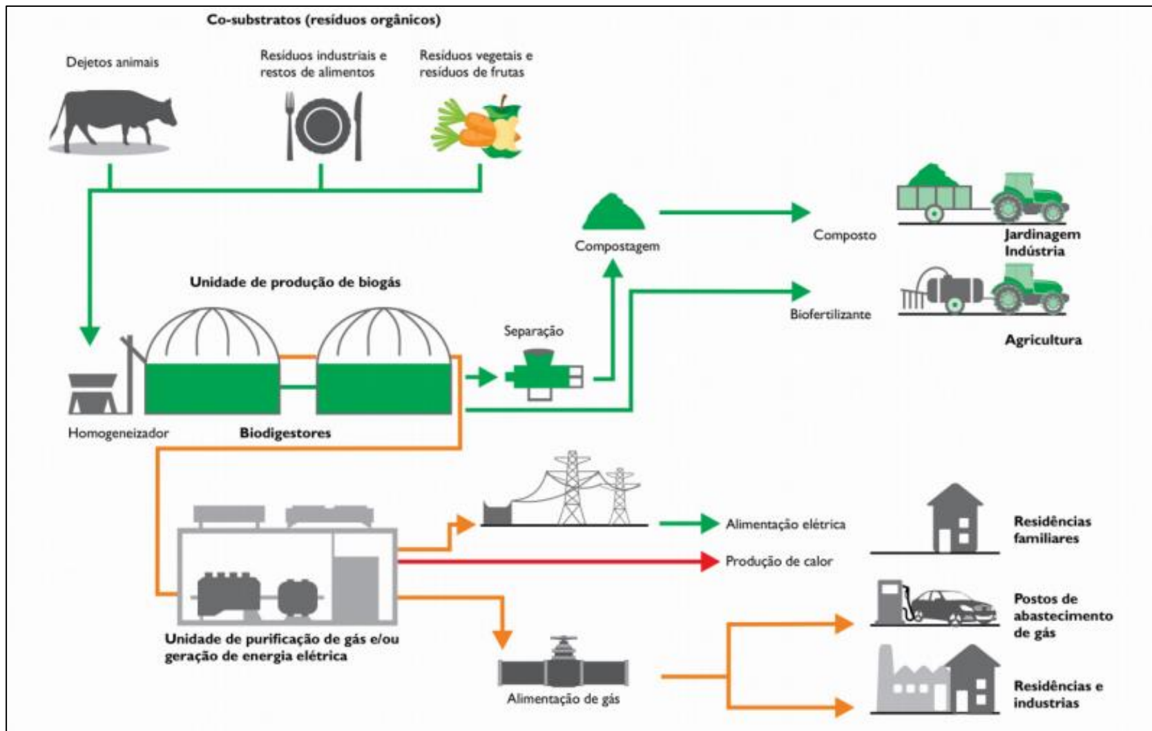
Figura 1. Sistema de transformação do biogás. Fonte: Atlas de Energias Renováveis, 2020.
